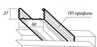
Потолочный профиль (ПП 60/27)
