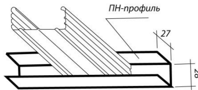
Потолочный направляющий профиль (ПН 28/27)
