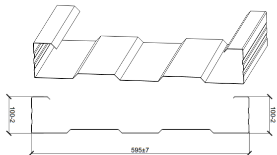
2. Сэндвич-профиль начальный
