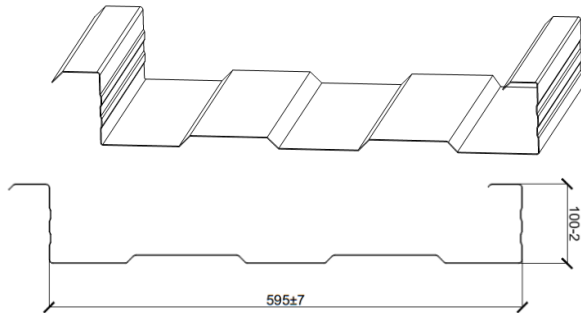
1. Сэндвич-профиль
