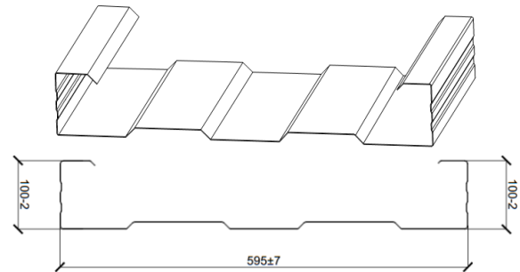
2. Сэндвич-профиль начальный
