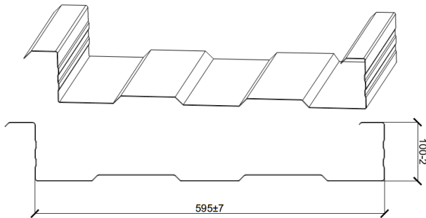
1. Сэндвич-профиль
