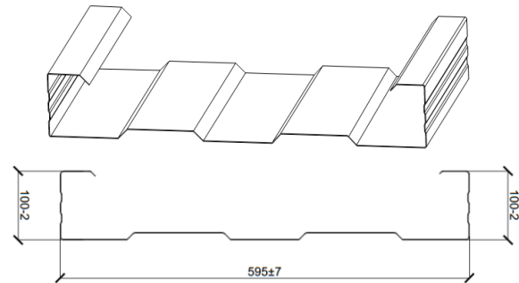
2. Сэндвич-профиль начальный
